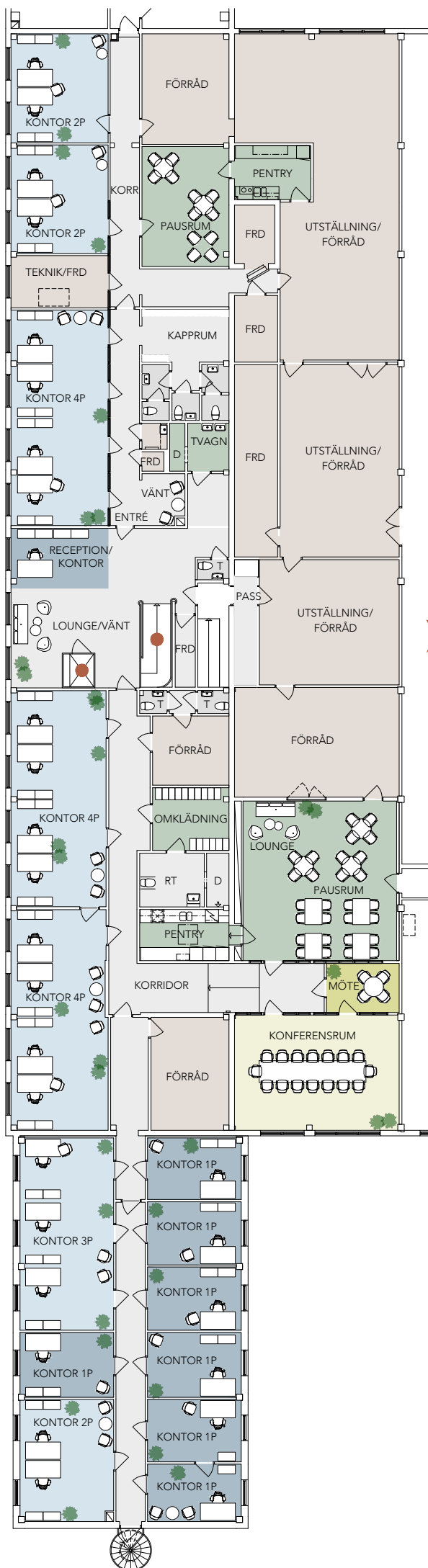
VÅNING 1, ENTRÉPLAN
